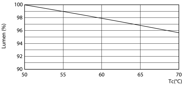
LEDtube 220-240V G13 2ft LumenVsTc
