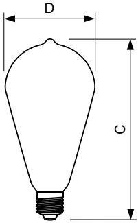
Bulb ST64 230V 7.5-48W 600lm 2000K E27
