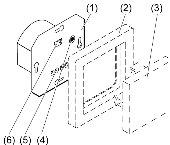
Afbeelding 1: Constructie apparaat
