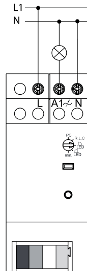
Afbeelding 3: Aansluitschema
