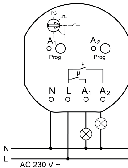
Afbeelding 2: Aansluitvoorbeeld
