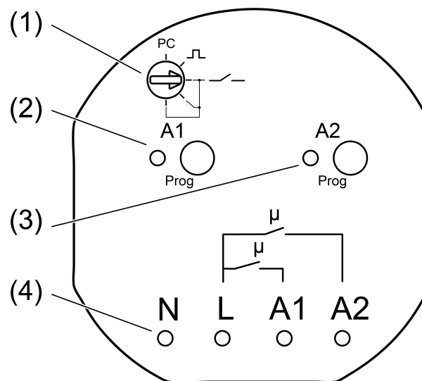
Afbeelding 1: Vooraanzicht
