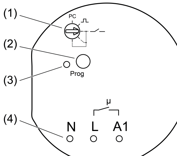
Afbeelding 1: Radiografische schakel-/knopactor
